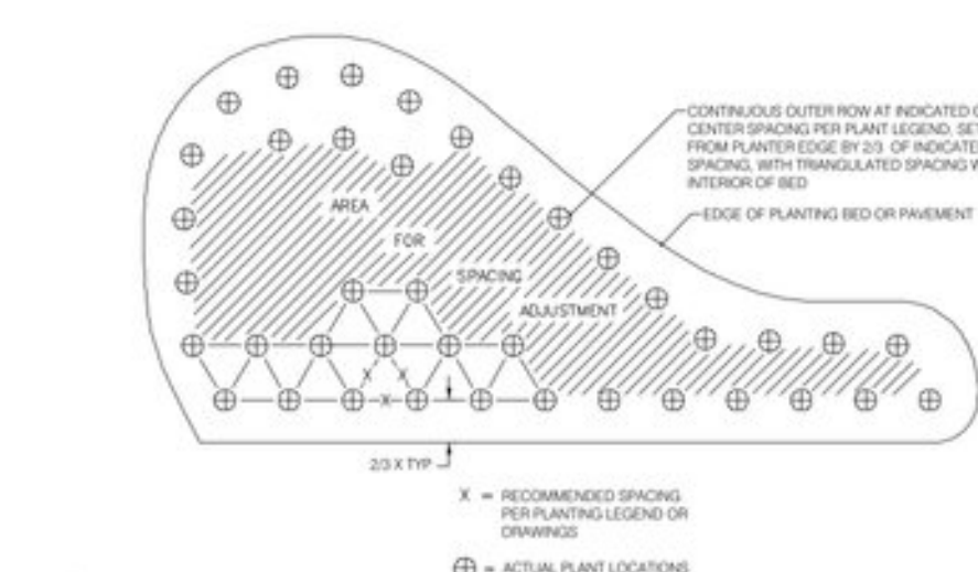
4 PLANTING LAYOUT SCALE: 1" = 1'-0"
